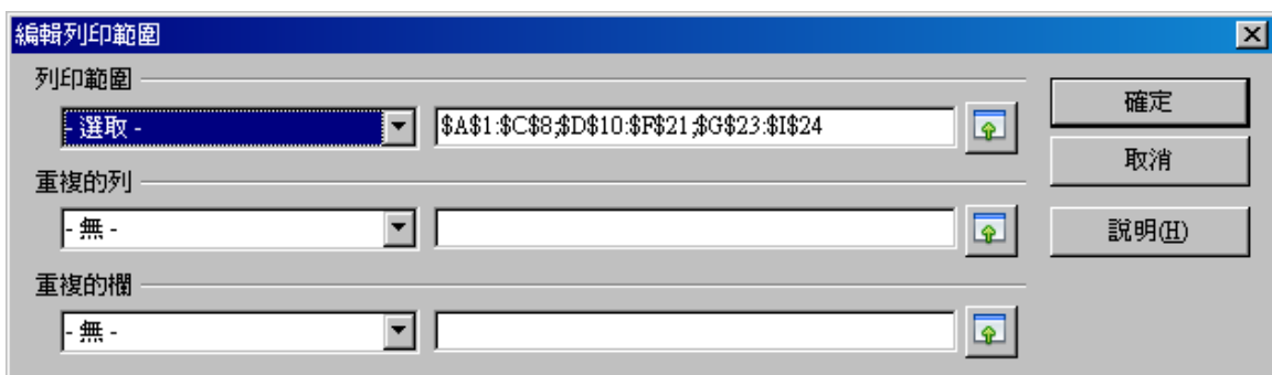
圖 5: 編輯列印範圍對話框
